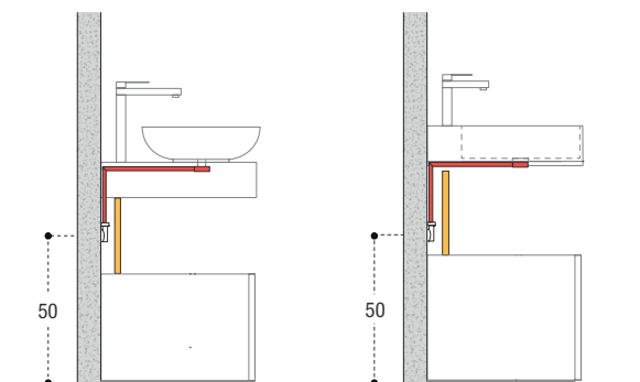
Posición del desagüe para encimera con lava- bo sobre encimera
