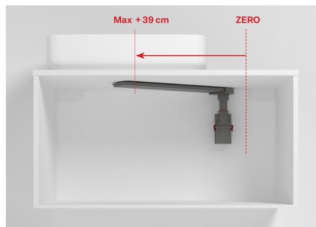
Posición con lavabo descentrado (Rotación máxima)
