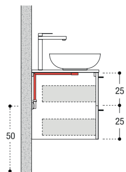
Posición del desagüe para mueble base con 2 cajones
