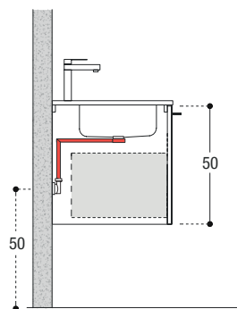
Posición del desagüe para mueble base con 1 gaveta
