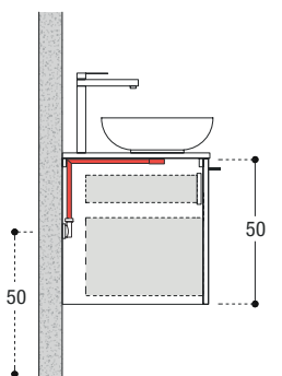
Posición del desagüe para mueble base con 1 gaveta y cajón interior
