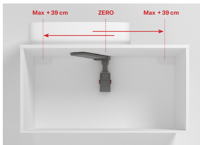
Posición con lavabo descentrado
